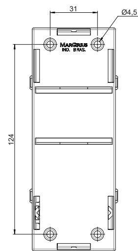
CP2 - CAIXA DE SOBREPÔR SLIM (MARGIRIUS)
