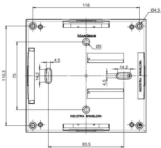
CP1 - CAIXA DE SOBREPÔR (MARGIRIUS)
